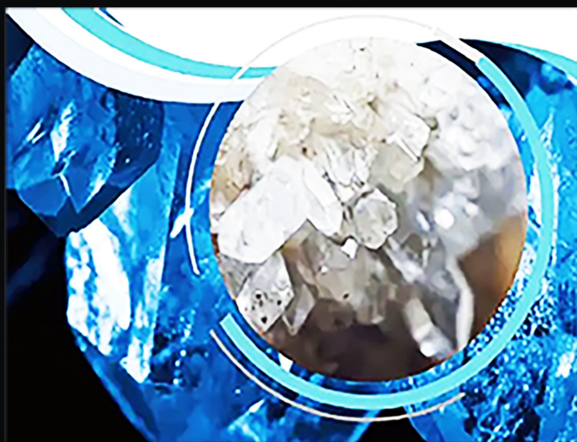
晶体生长
